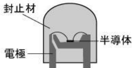
LEDの構造
